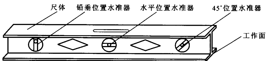
图 3 铝制的水平尺
