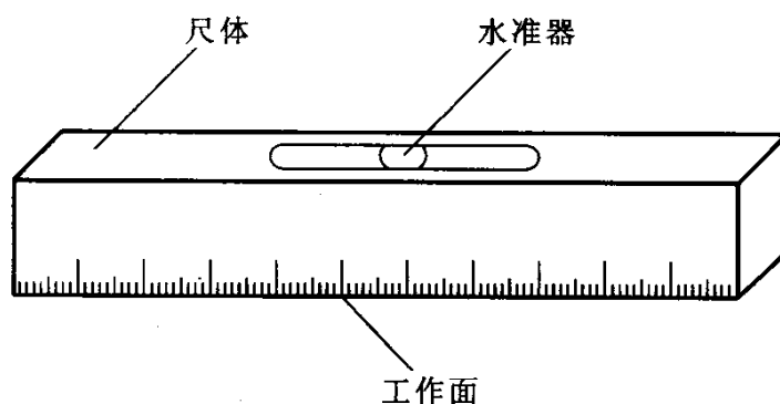
图 2 木制的水平尺
