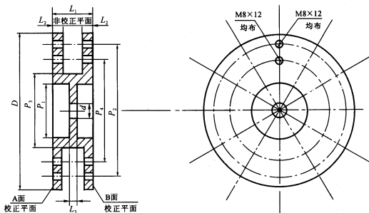
图 A1 校验转子形状示意图
