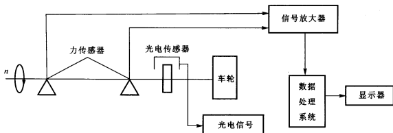
图1 平衡机原理示意图
